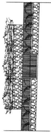
PROSPETTO SUD - OVEST Scala 1:100
